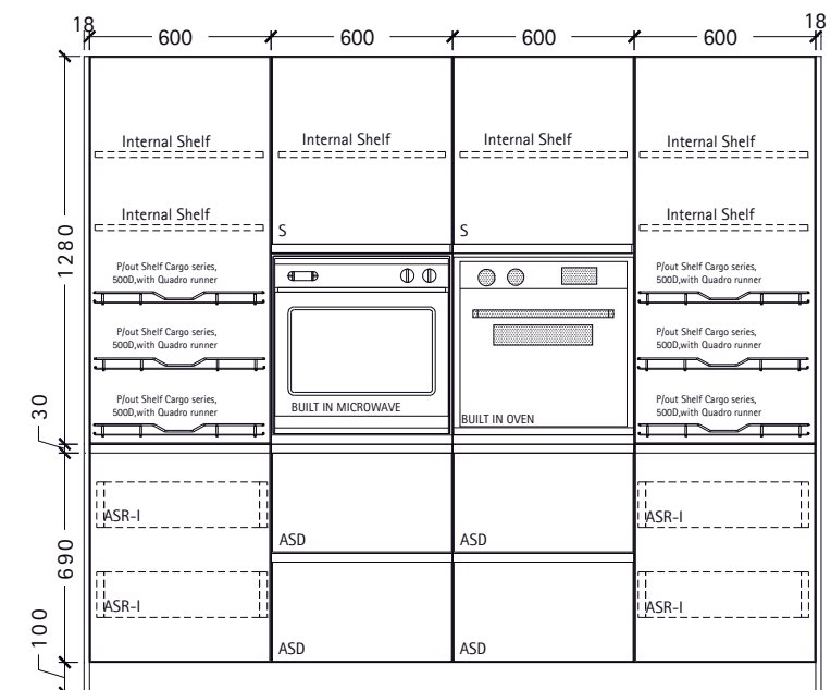
Elevation B
