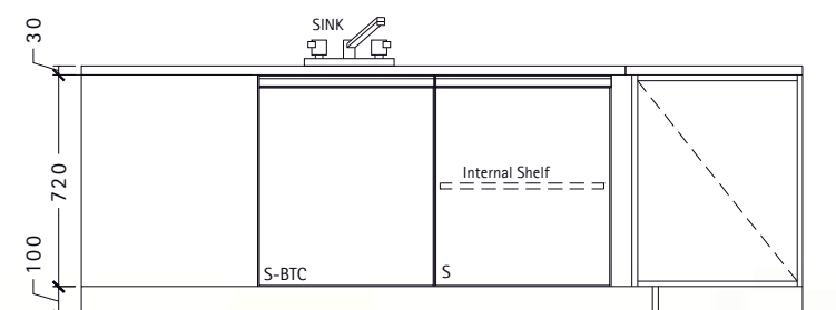
Elevation B
