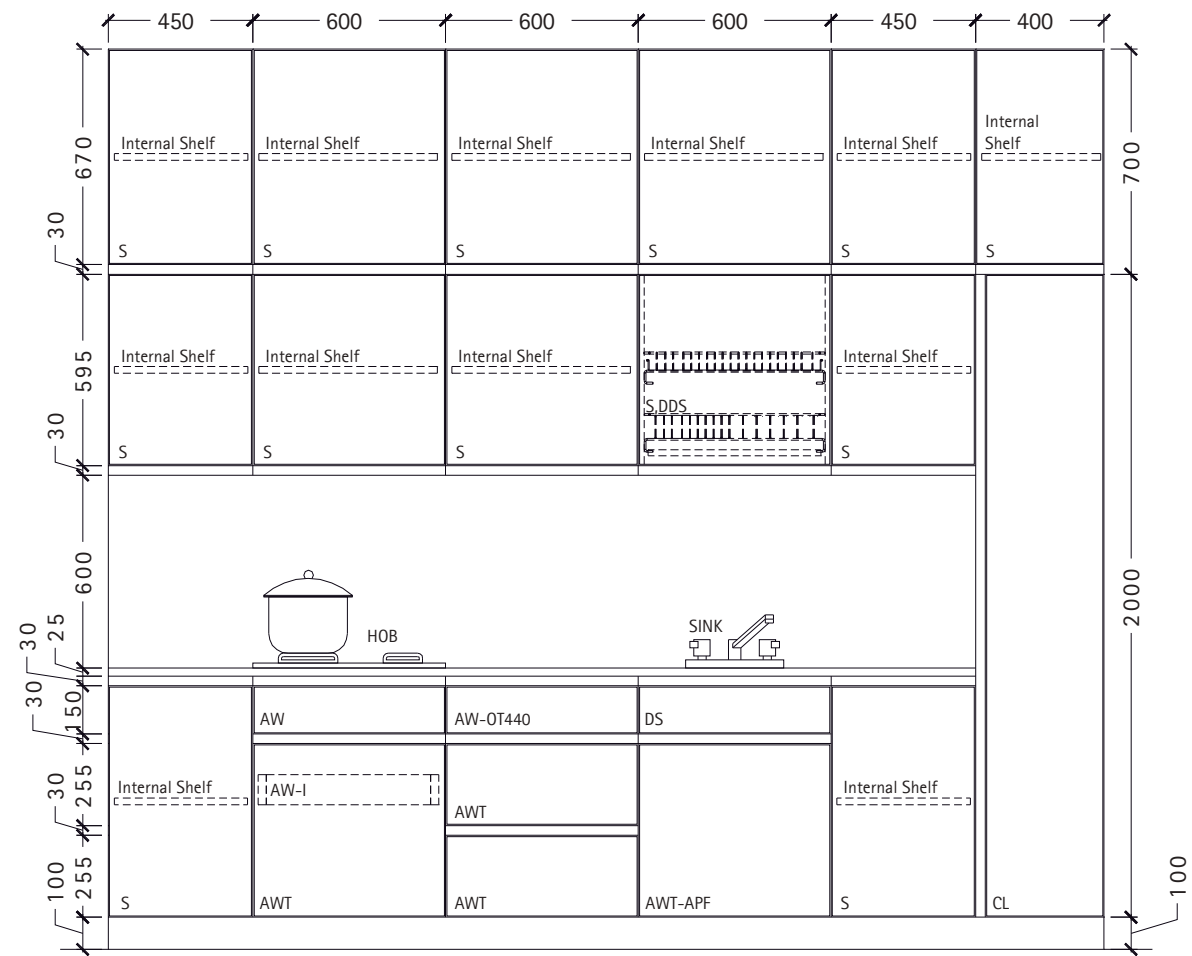
Elevation A
