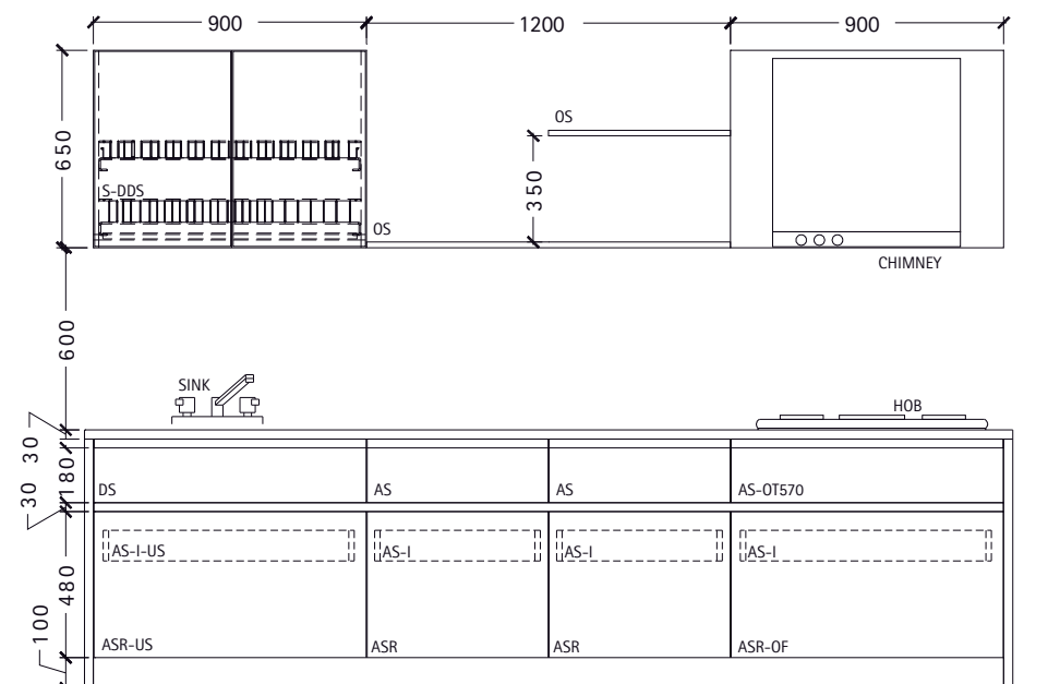
Elevation A
