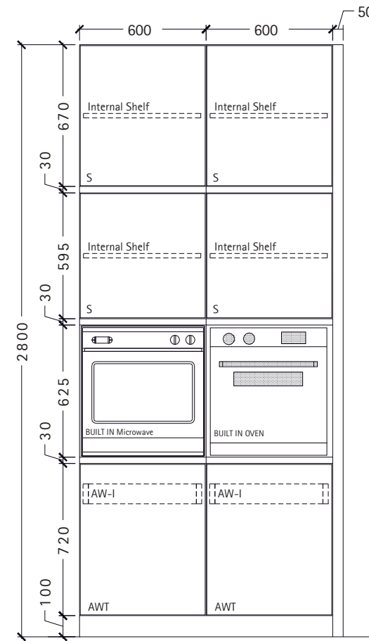
Elevation B
