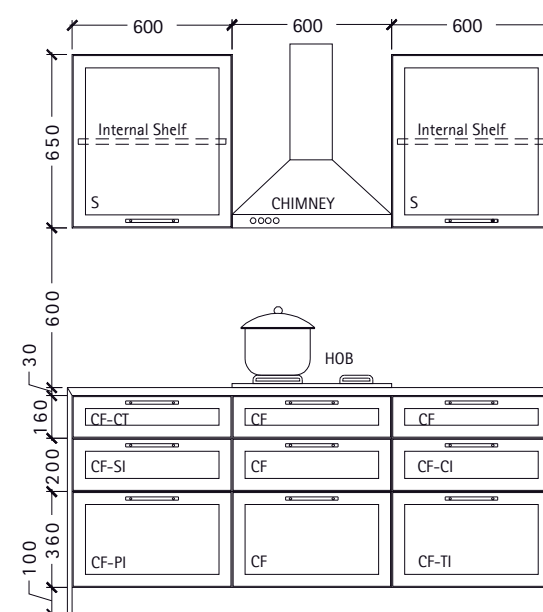
Elevation B
