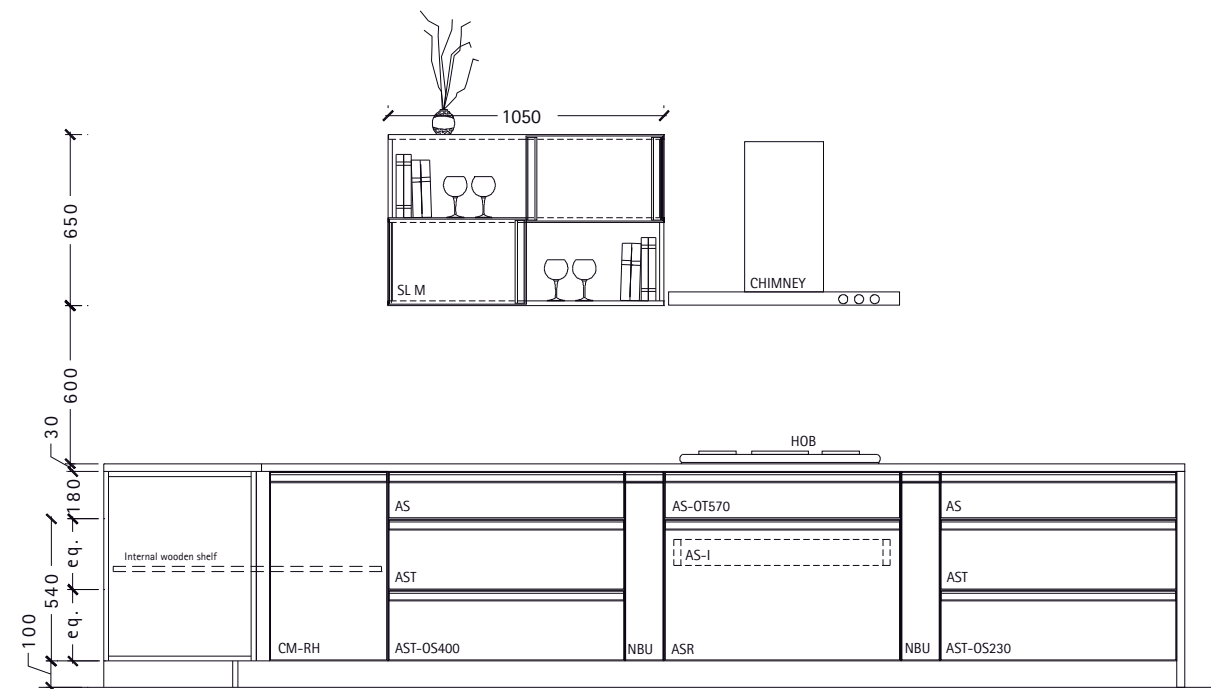
Elevation A
