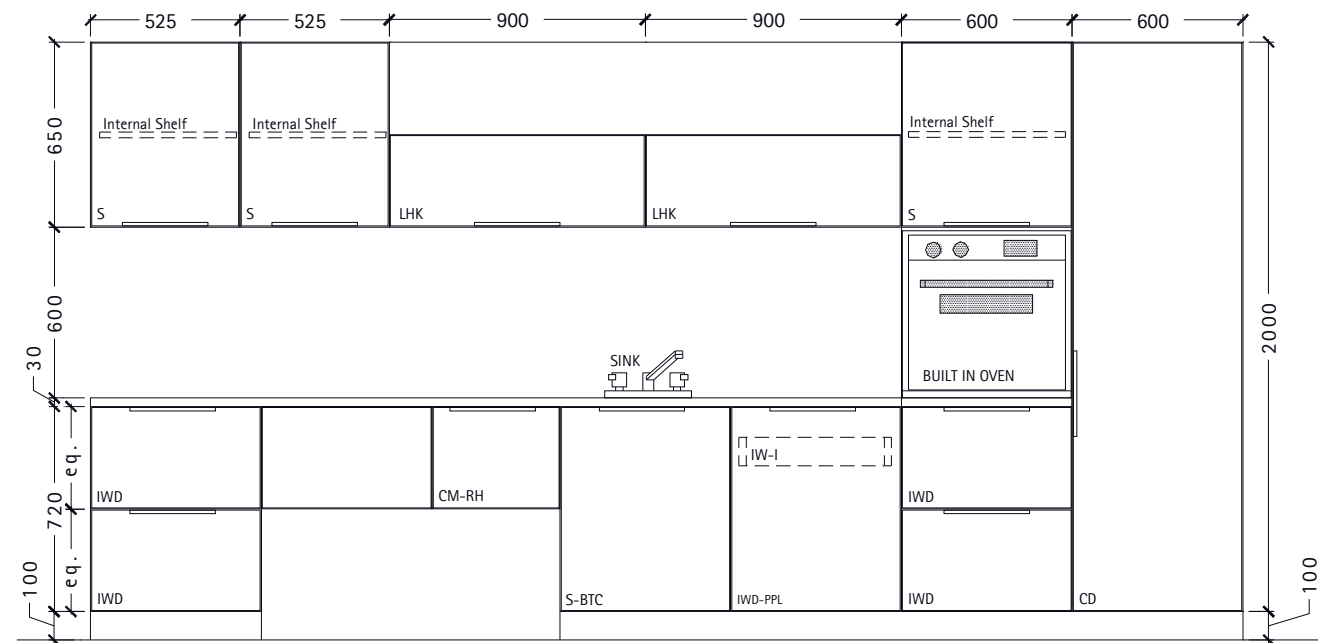
Elevation A
