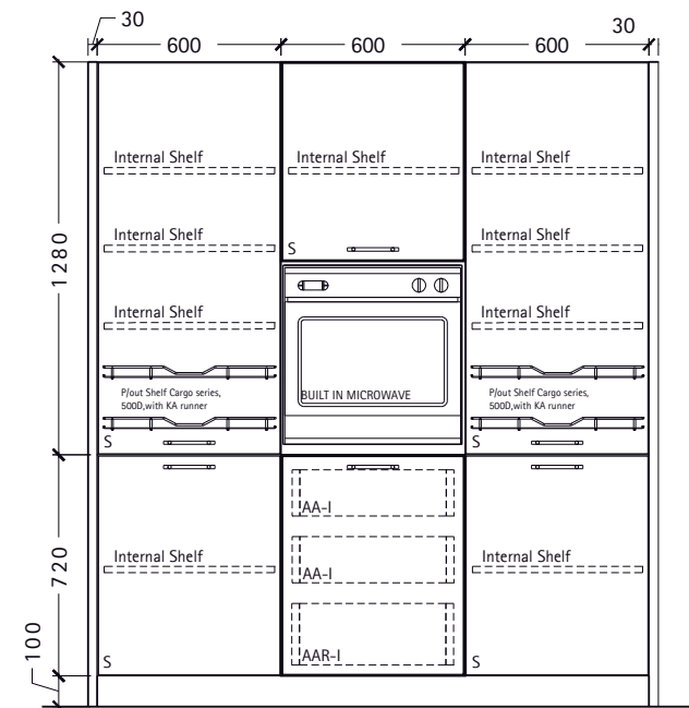
Elevation B
