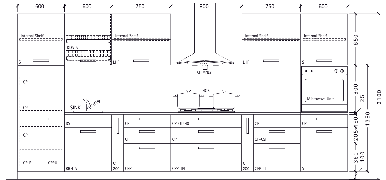
Elevation
