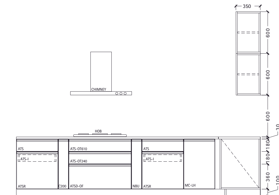
Elevation B
