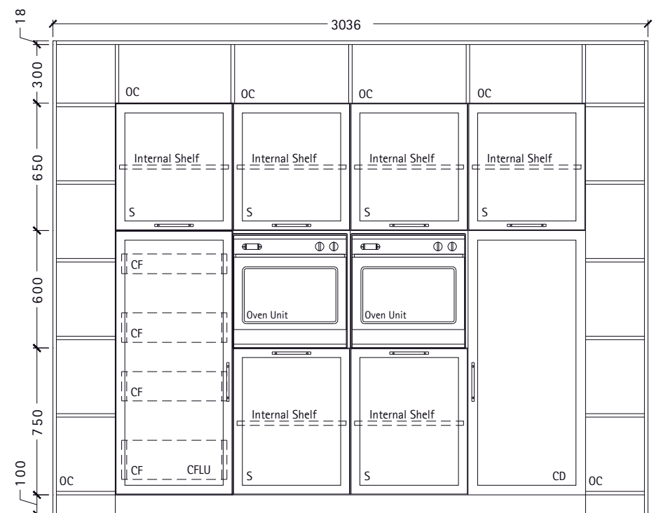
Elevation A
