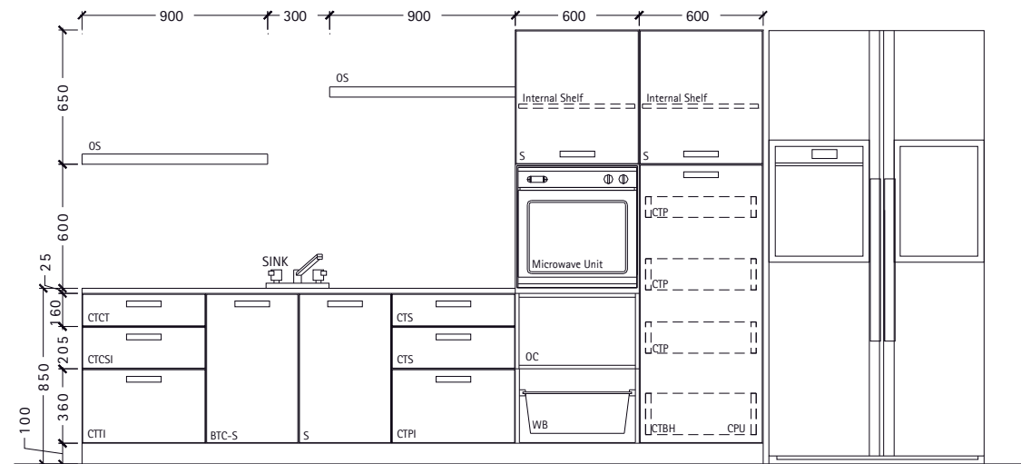
Elevation A
