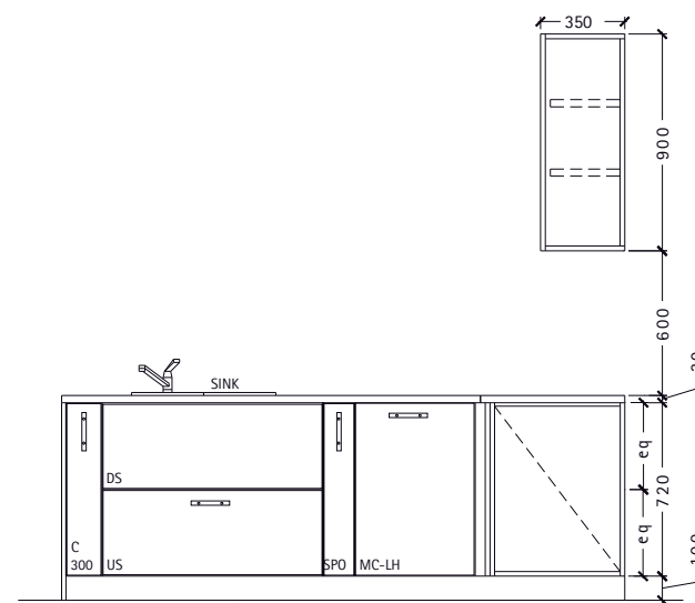
Elevation B
