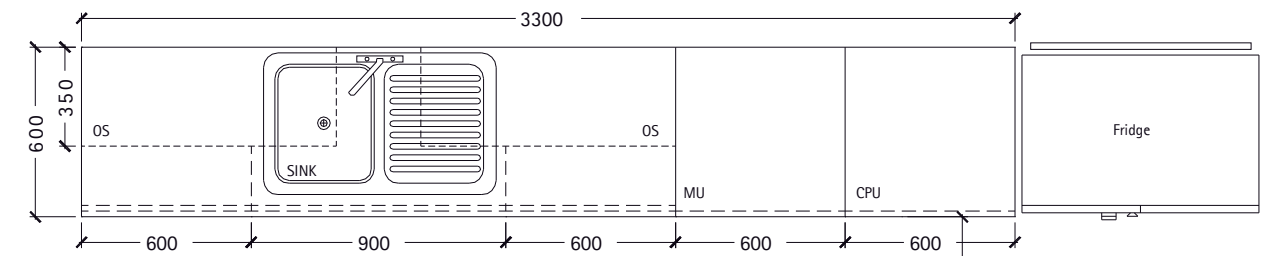
Elevation B
