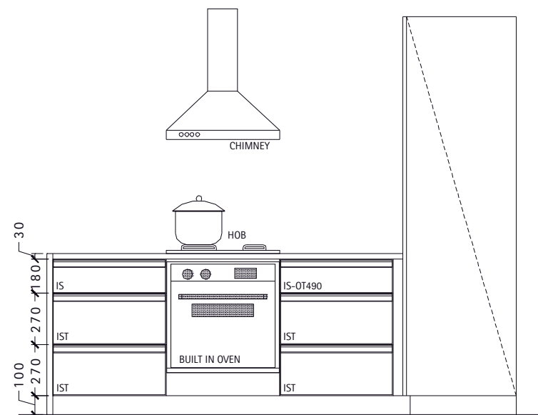
Elevation A
