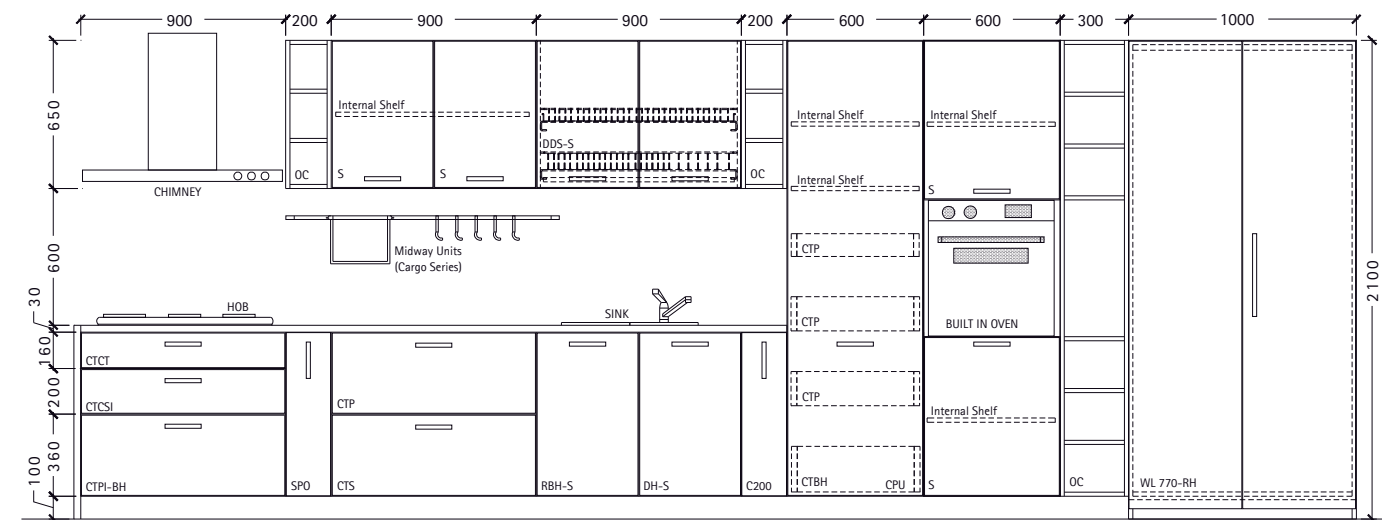
Elevation
