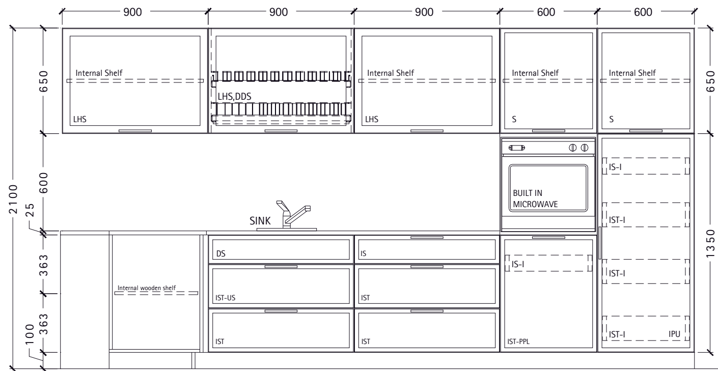
Elevation A
