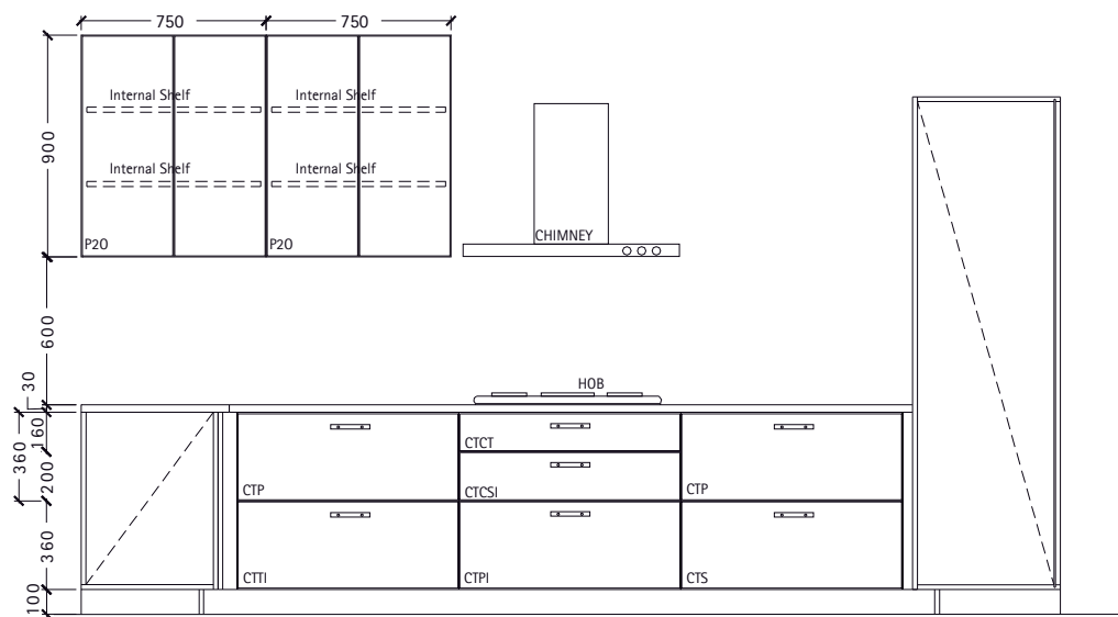
Elevation A
